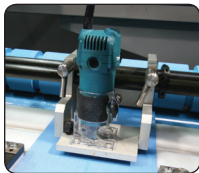
GRINDER
